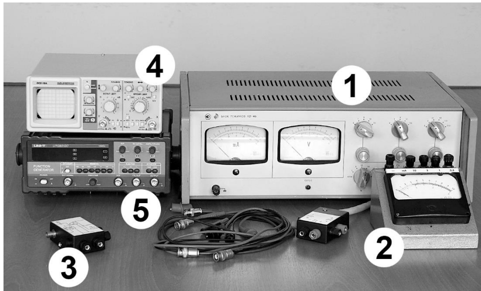
Рис. 4.1. Внешний вид лабораторной установки.
