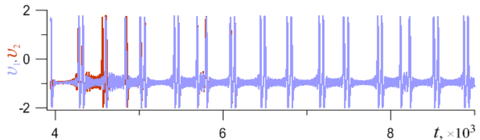
Рис. 2.2. Установление полной синхронизации колебаний
