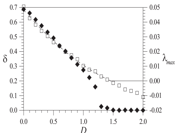
Рис. 3.2. Зависимость относительной ошибки синхронизации \delta (символы «◆») и старшего ляпуновского показателя \lambda_{max} (символы «□») от интенсивности шума D
